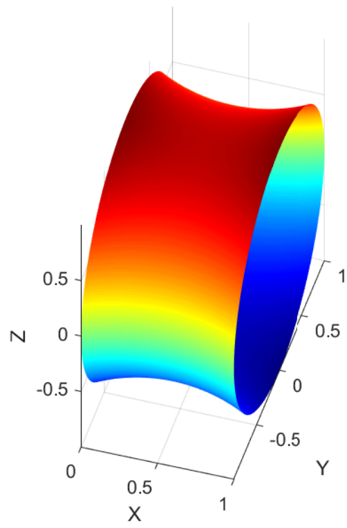
Sólido de revolución ( n=50 , t_k=0.01 )
